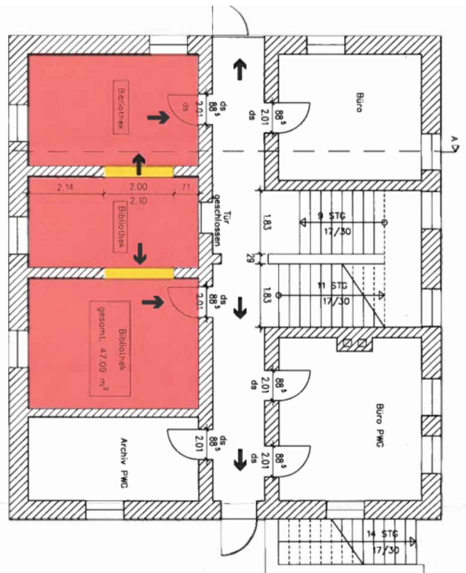
Grundriss Erdgeschoss
