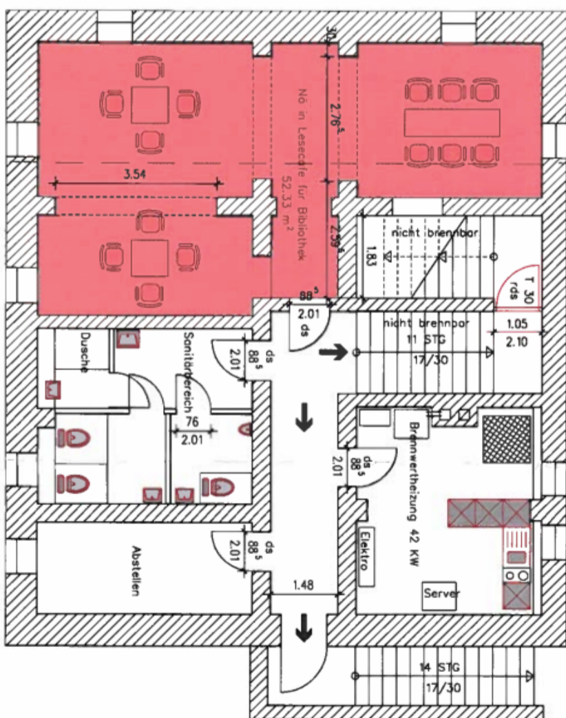
Grundriss Kellergeschoss
